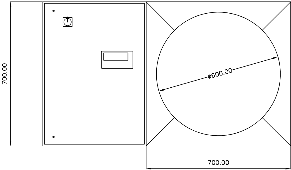
VOORAANZICHT
