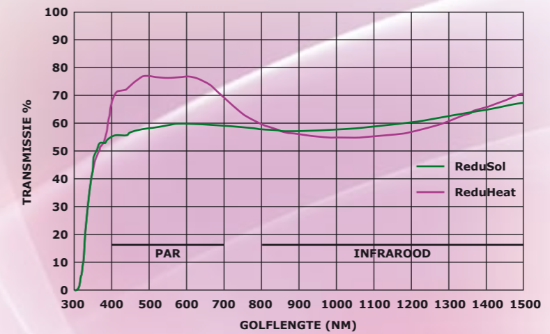
VERGELIJKING TRANSMISSIESPECTRA REDUSOL EN REDUHEAT
